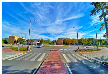
■ Kecskemét , Nyíri út-Akadémia krt. kereszteződés térségének átalakítása és a Bács-Kiskun Megyei Kórházi körforgalmú csomópont tervezése (2021)
